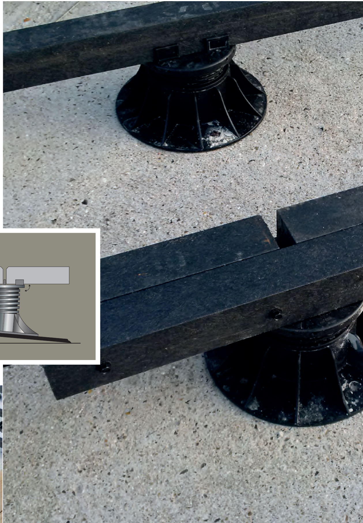
⬆ Самовирівнювальна регульована опора
