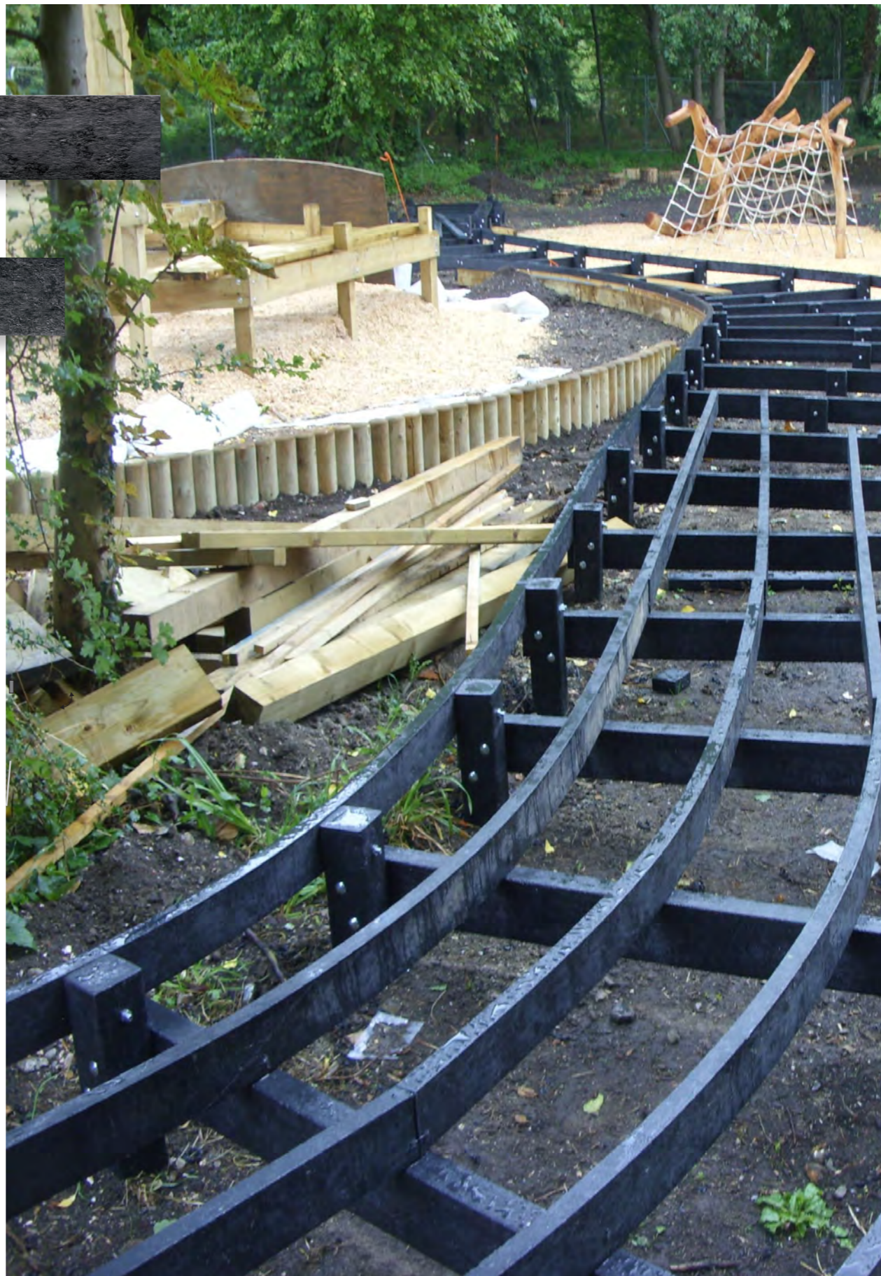
Кріплення для каркасу 6,3 x 90 мм.
