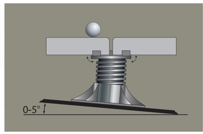
⬆ Самовирівнювальна регульована опора
